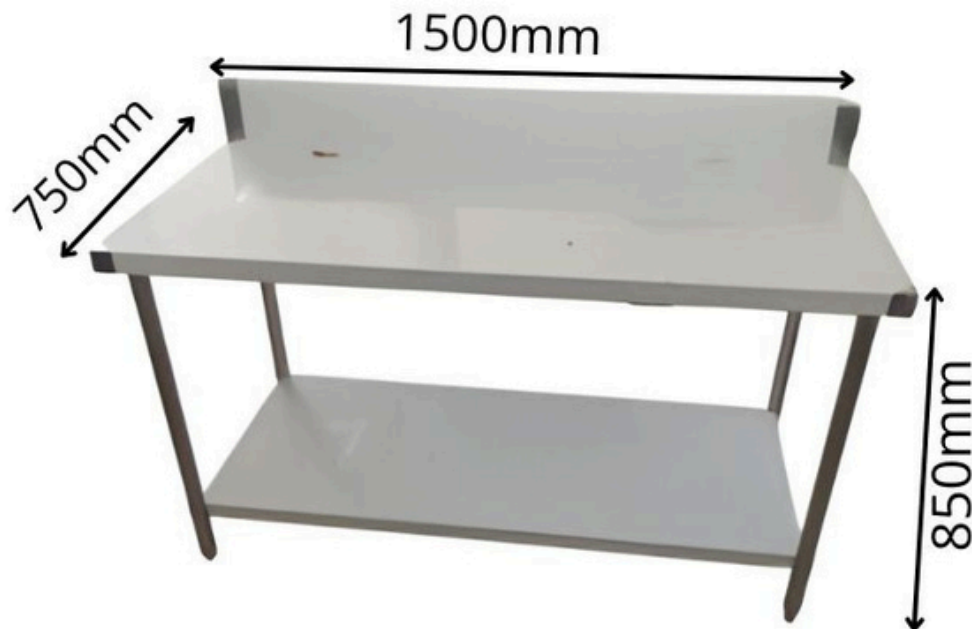
MESA DE TRABAJO AC/INOX CON TOPE Y UNA REPISA 1500X700X850 Modelo: WTF-215S Codigo: 009005243
